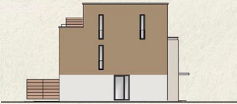
Seitenansicht (Endhaus)
